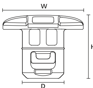
Element mocujący, wciskany T50RPBM9 (zestaw)
